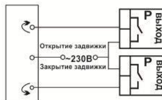
Подключение электрозадвижки
