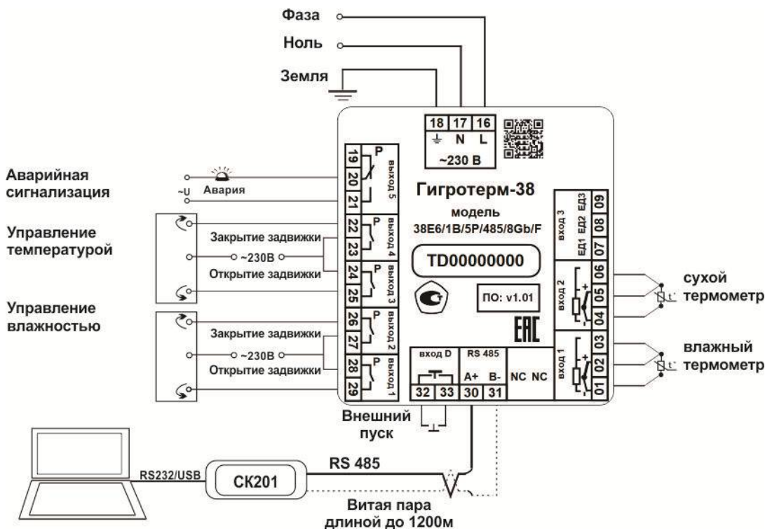
Рисунок 7 – Схема подключения прибора
