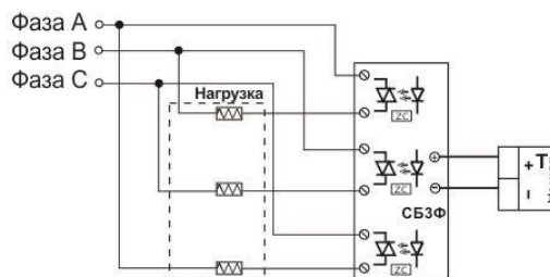
Подключение трехфазной нагрузки в шестипроводной схеме
