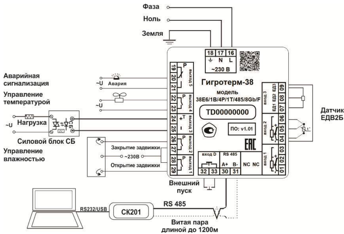
Рисунок 6 – Схема подключения прибора
