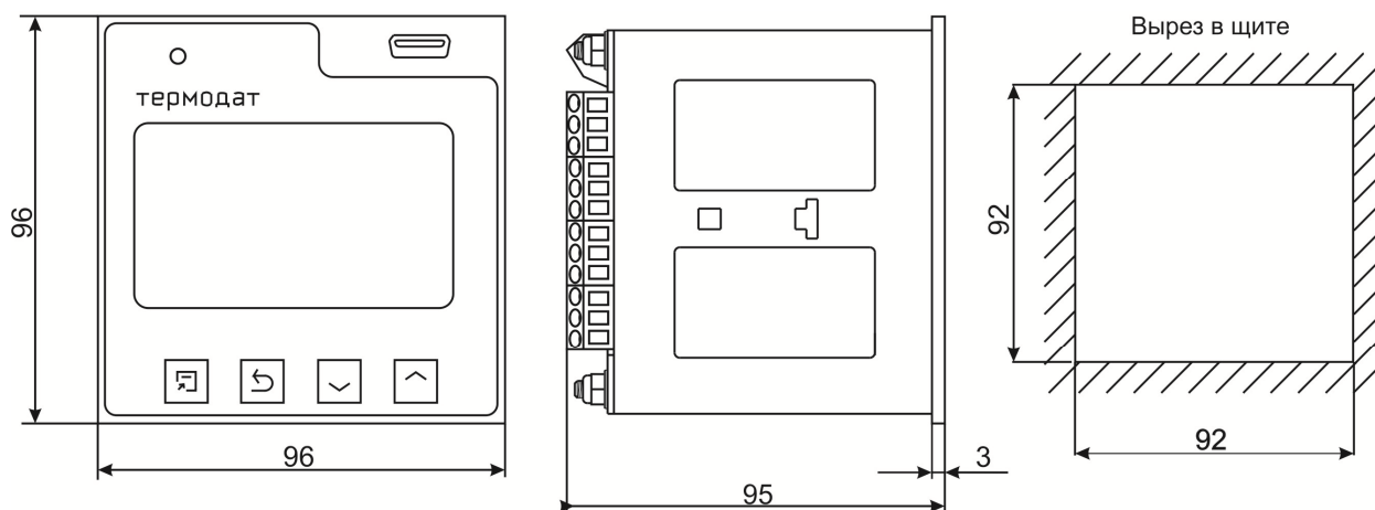
Рисунок 8 – Габаритные размеры прибора Гигротерм-38Е6/...../(F)
